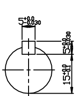
INPUT SHAFT
